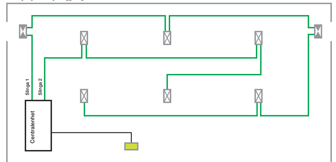
Exempel på kabelförläggning inom en brandcell.
